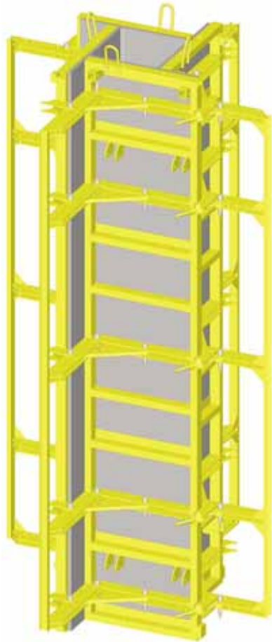
Grip Stützenschalung 340cm Art.-Nr.: 170.006.1000 Gewicht: 750,0 kg
