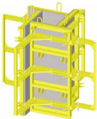
Grip Stützenschalung 150cm Art.-Nr.: 170.006.1002 Gewicht: 400,0 kg
