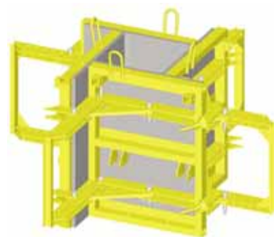
Grip Stützenschalung 90cm Art.-Nr.: 170.006.1003 Gewicht: 265,0 kg
