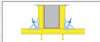
Unterzug mit vertikalen H20 Trägern
