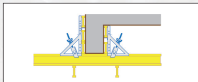
Randunterzug mit Deckenanschluss
