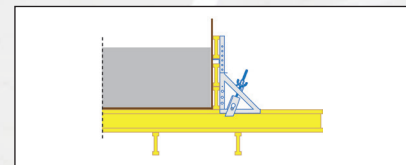
Deckenrandschalung
